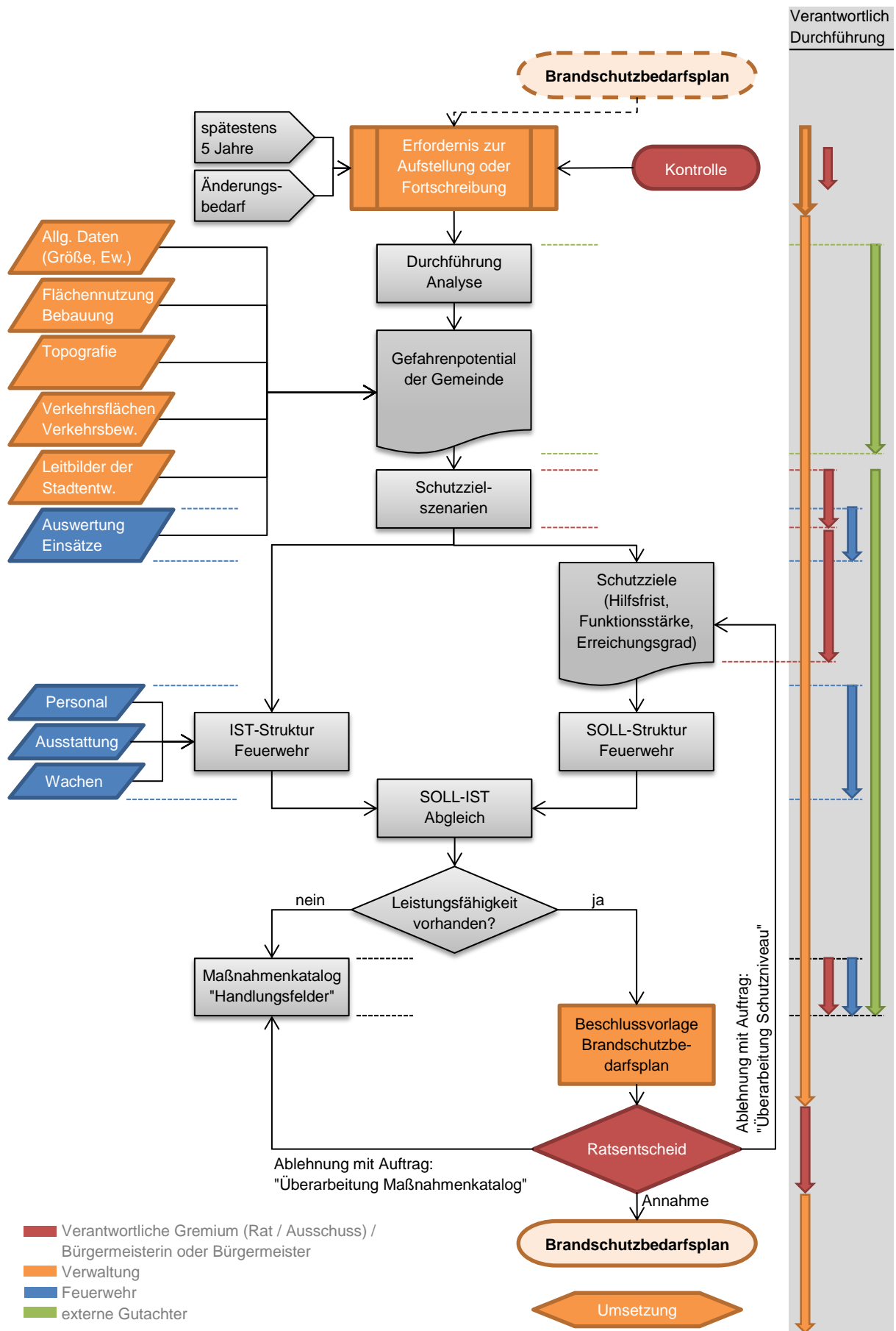
Abbildung 1 Ablaufdiagramm Brandschutzbedarfsplanung
